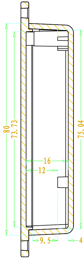
SEC A-A
