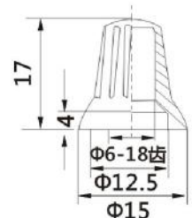
KA483-5型 Plastic Knob
